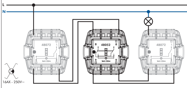
PERMUTATEUR LUMINEUX
