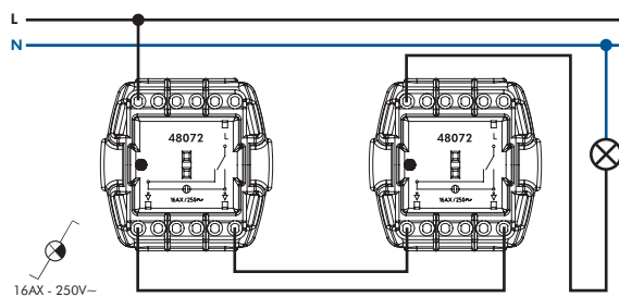
VA-ET-VIENT LUMINEUX
