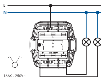
VA-ET-VIENT LUMINEUX
