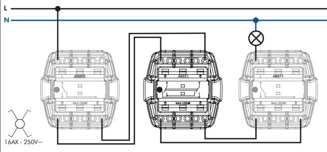
PERMUTATEUR
