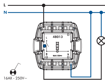
INTERRUPTEUR TÉMOIN
