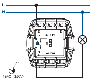
INTERRUPTEUR LUMINEUX
