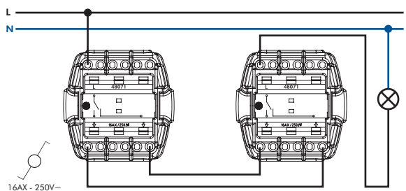
VA-ET-VIENT
