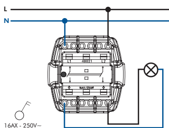
VA-ET-VIENT
