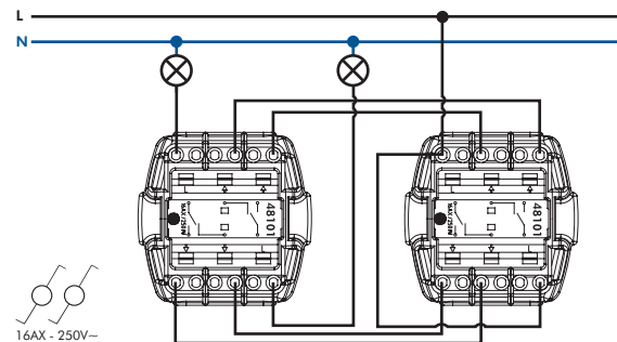
VA-ET-VIENT DOUBLE - 10A ET 20A
