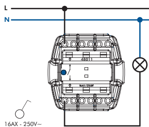
INTERRUPTEUR UNIPOLAIRE
