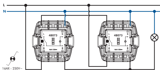
VA-ET-VIENT TÉMOIN
